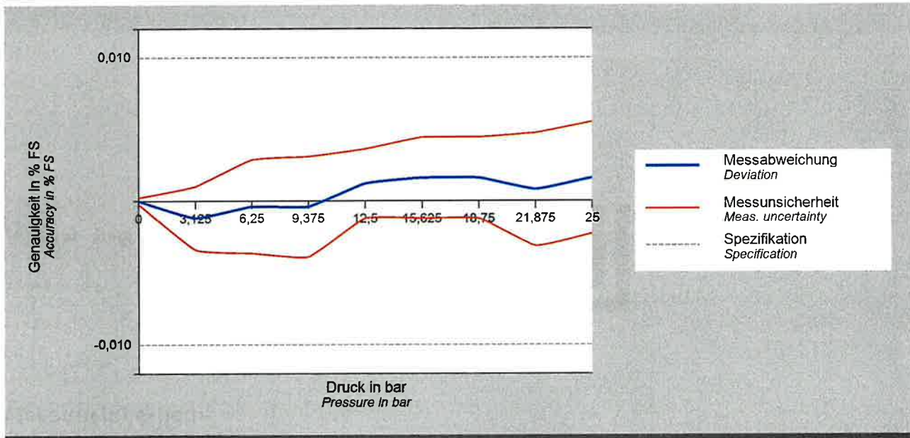
Grafische Darstellung der Messunsicherheit Graphical representation of measurement uncertainty
